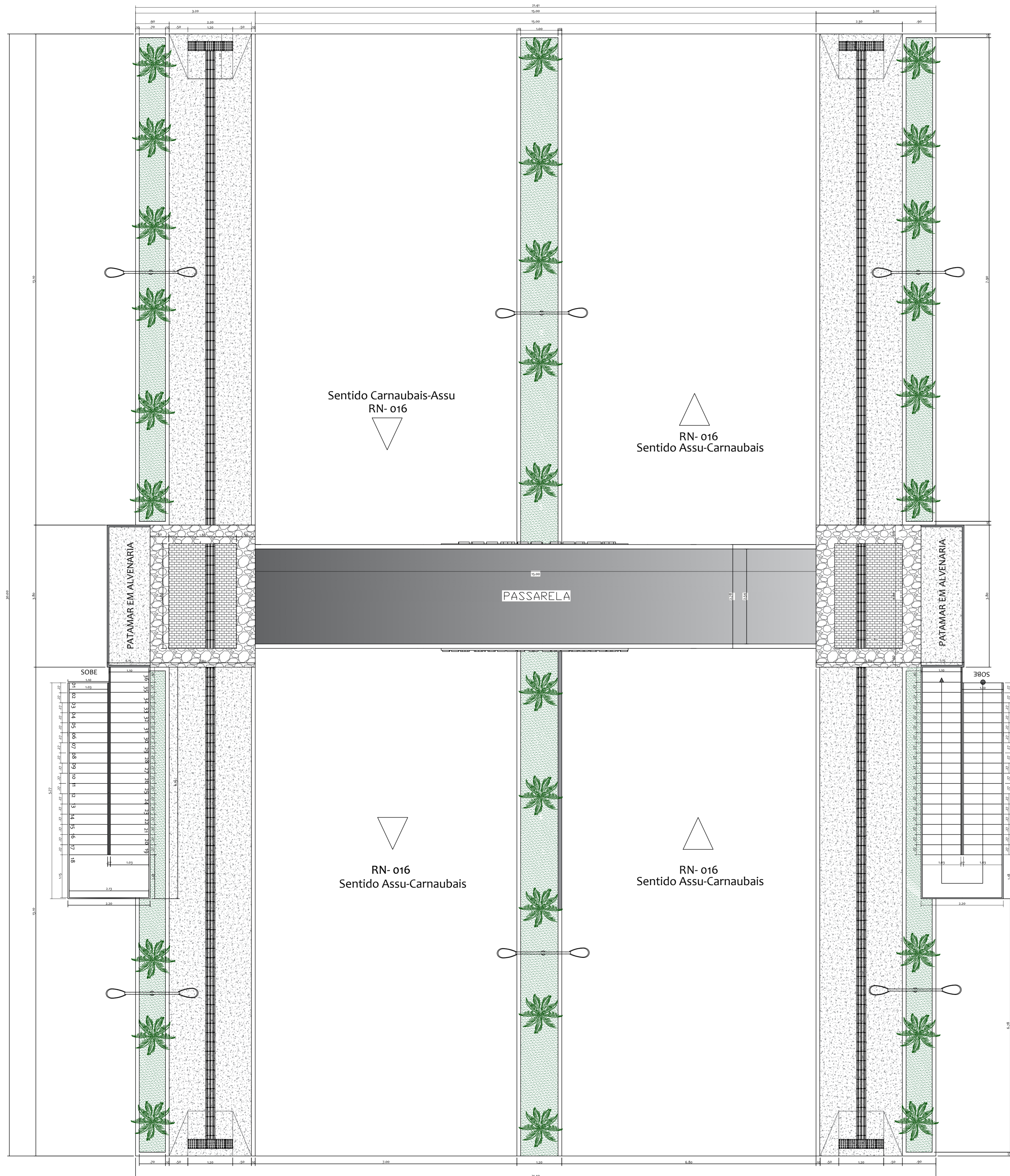
PLANTA BAIXA DO PÓRTICO Construção de um pórtico na cidade de Carnaubais/RN Escala: 1/50
